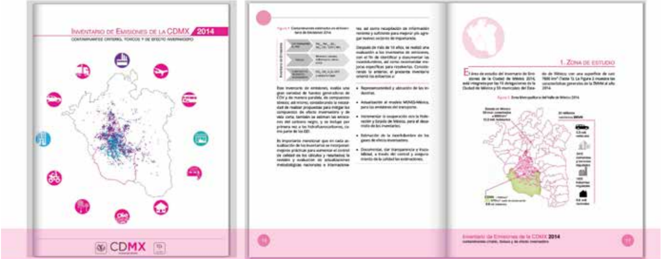
INVENTARIO DE EMISIONES DE LA CDMX 2014 (SE REALIZA POR NORMA CADA 2 AÑOS)
